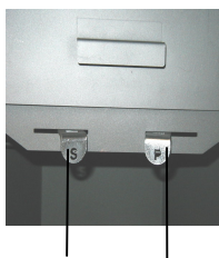
Regulador del aire secundario (S) Regulador del aire primario (P)
