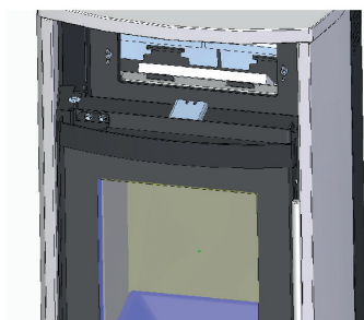
Katalysator hinter dem Teefach (weiß in der Abbildung)
