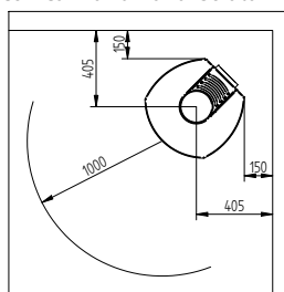
Distanza da materiali infiammabili senza canna fumaria isolata
