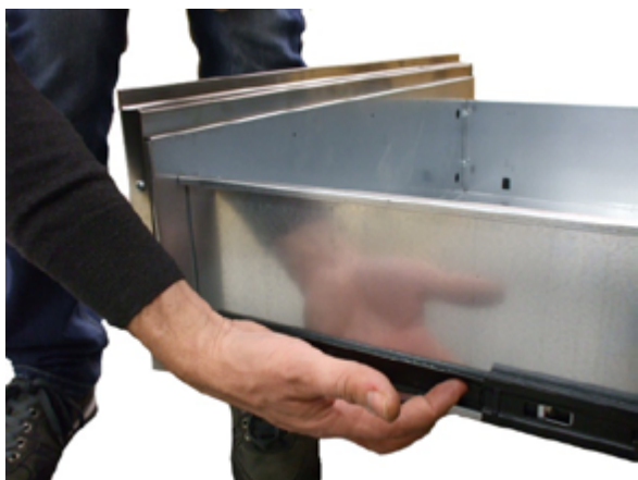
Fig. 26 - Führung aushaken
