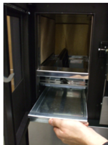
Fig. 25 - Den Aschenkasten entnehmen
