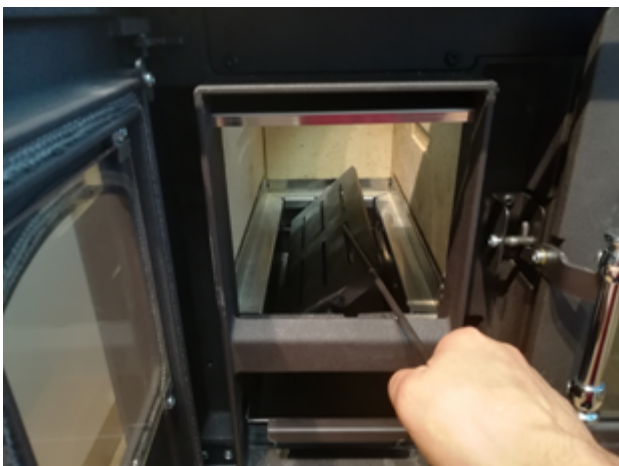
Fig. 24 - Rost herausziehen
