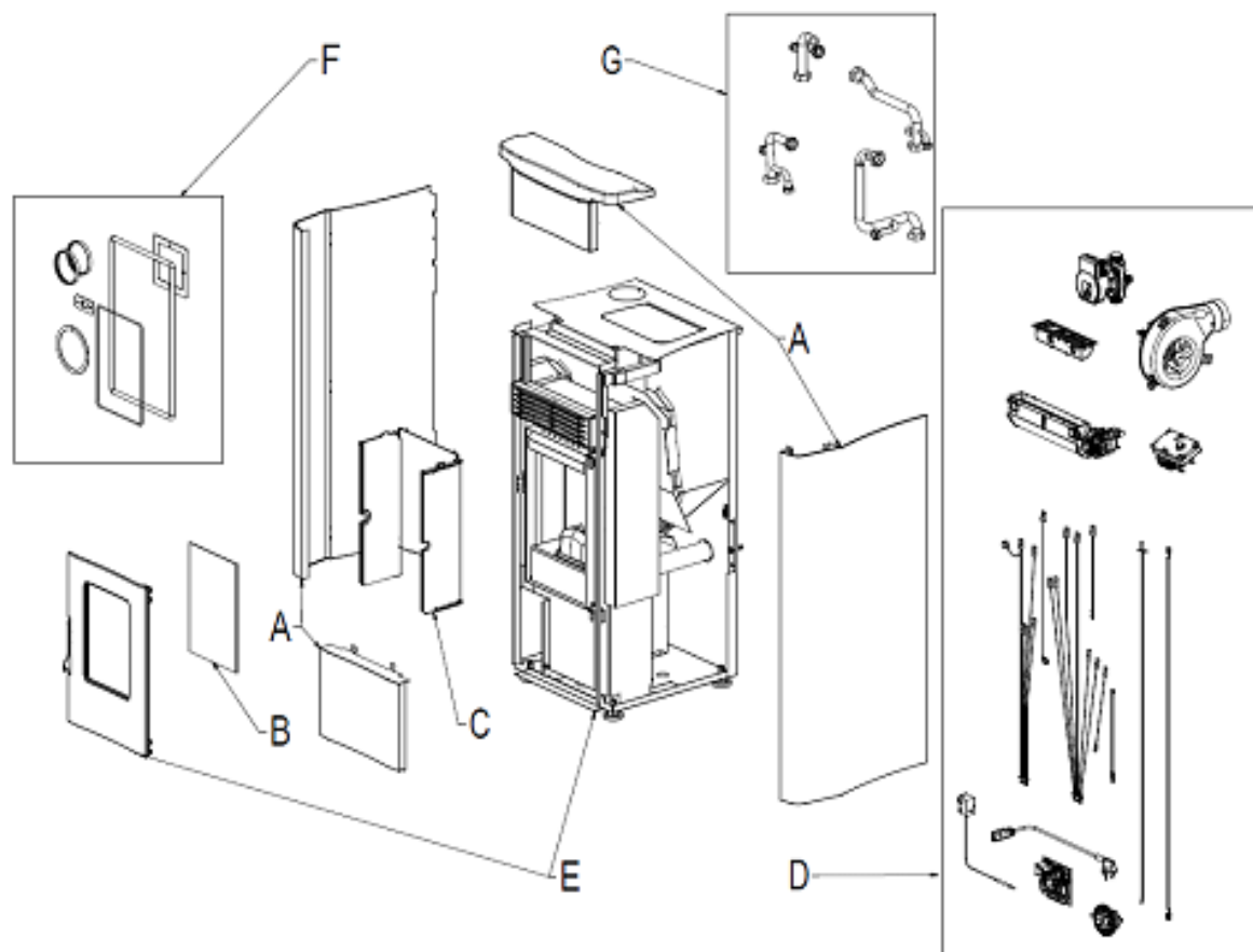
Fig. 2 - Explosionszeichnung
