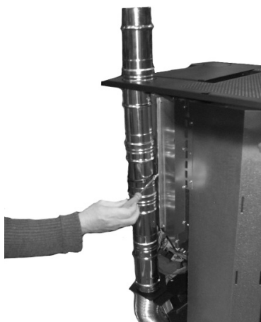
Fig. 56 - Positionierung der Rohre für oberen Kanal
