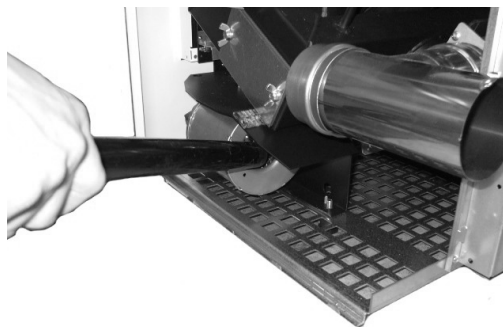
Fig. 107 - Reinigung Raumventilator
