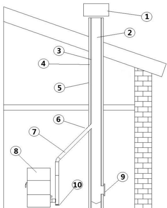
Fig. 6 - Bauteile Kamin
