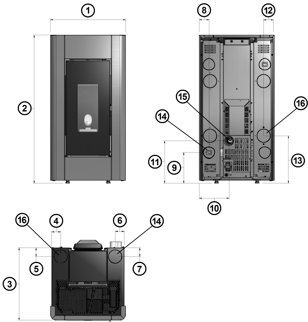
Fig. 19 - Allgemeine Abmessungen: Prince³ / Prince³ Plus
