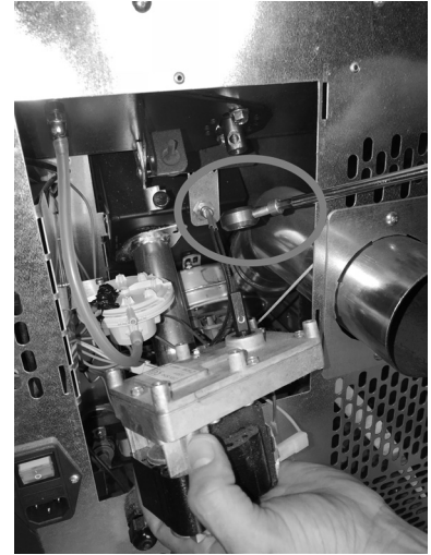
Fig. 72 - Getriebemotor entfernen
