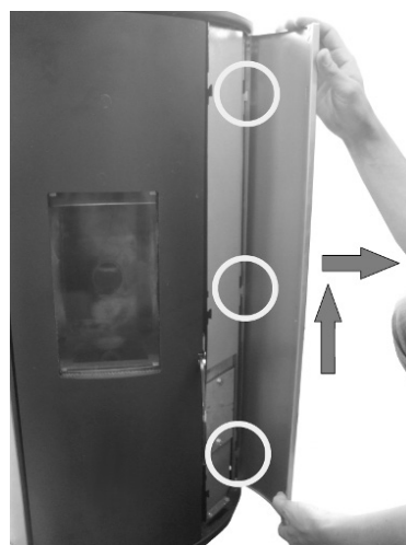
Fig. 80 - Sfera 3 / Sfera 3 Plus: Die Seitenplatten auslösen
