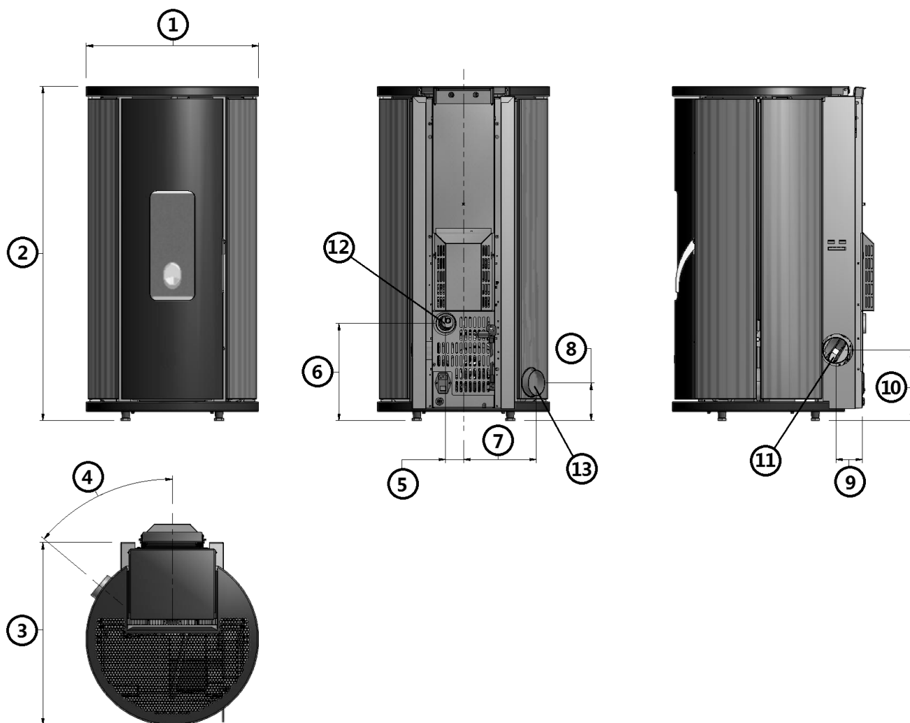
Fig. 18 - Allgemeine Abmessungen: Sfera³ / Sfera³ Plus / Globe
