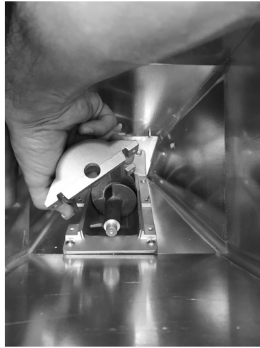
Fig. 71 - Gehäuse entfernen
