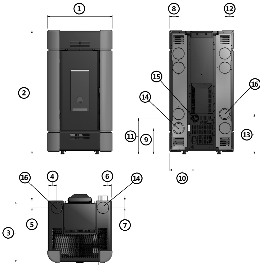
Fig. 16 - Allgemeine Abmessungen: Sire³ Plus
