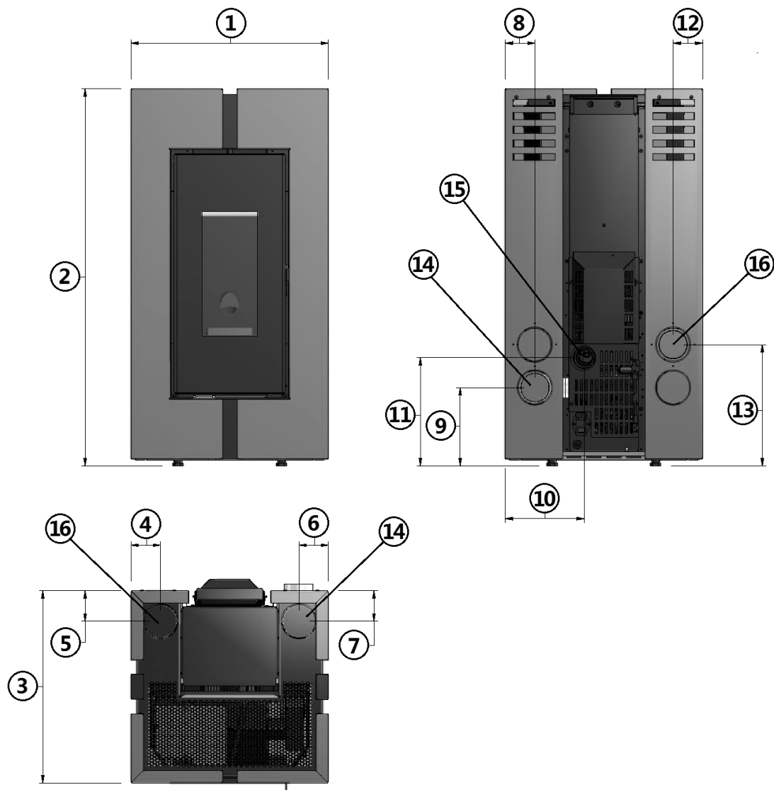
Fig. 17 - Allgemeine Abmessungen: Doge³ Plus
