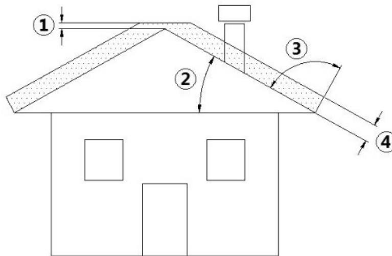
Fig. 3 - Geneigtes Dach
