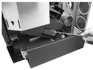
Fig. 100 - Reinigung mit Flaschenbürste 2
