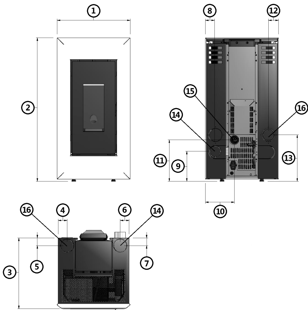
Fig. 15 - Allgemeine Abmessungen: Vega / Trend
