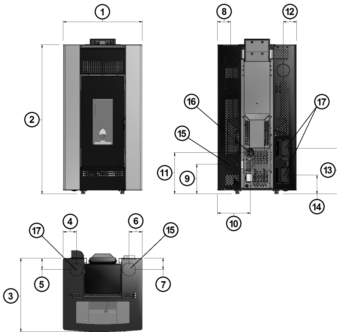
Fig. 22 - Allgemeine Abmessungen: Joy At
