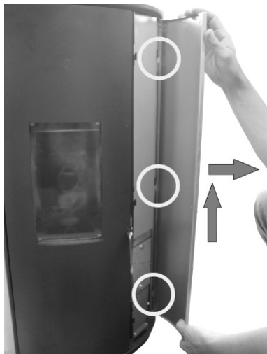
Fig. 36 - Montage Platten
