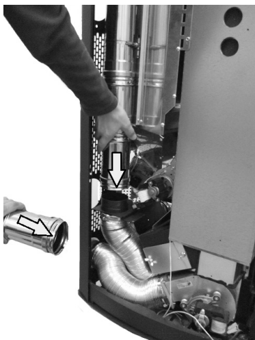
Fig. 63 - Positionierung der Rohre für Kanalisierung
