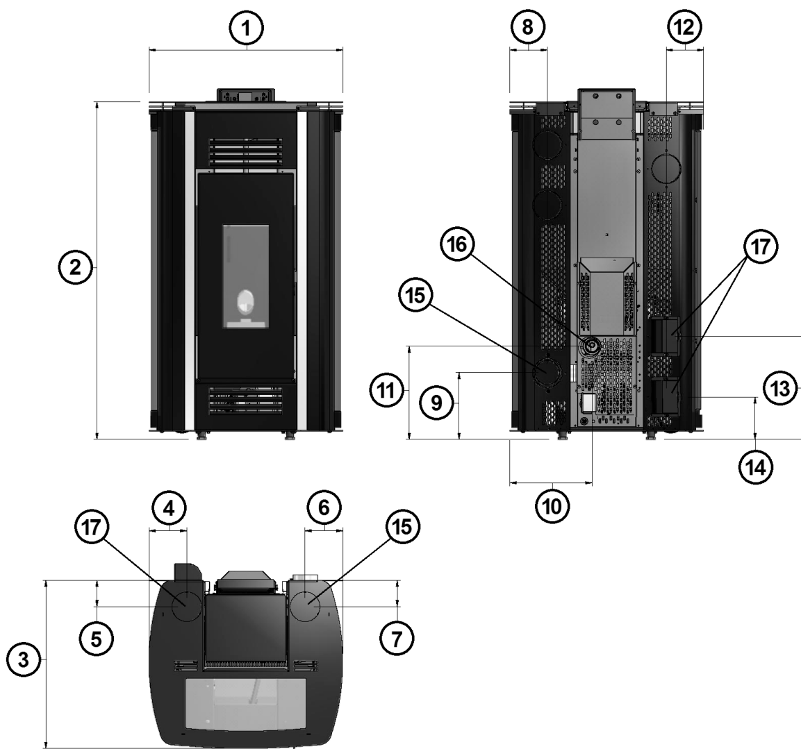
Fig. 21 - Allgemeine Abmessungen: Venus³ Plus 12,5KW
