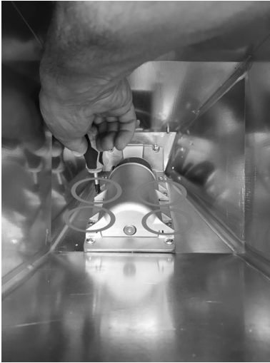
Fig. 70 - Lösen der Schrauben
