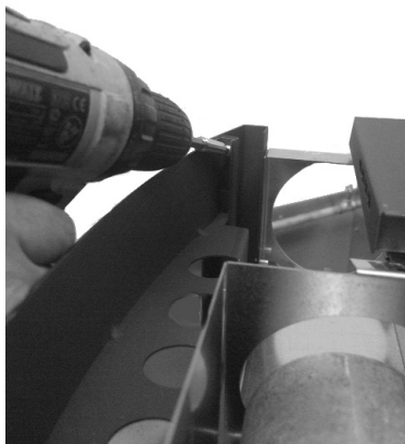
Fig. 44 - Entfernen der oberen gebogenen Profile
