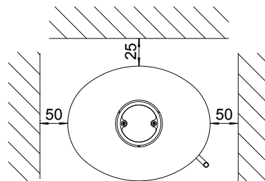
Poêle installé droit dans le coin
