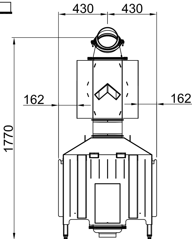
~1:20 Thermobox, breit
